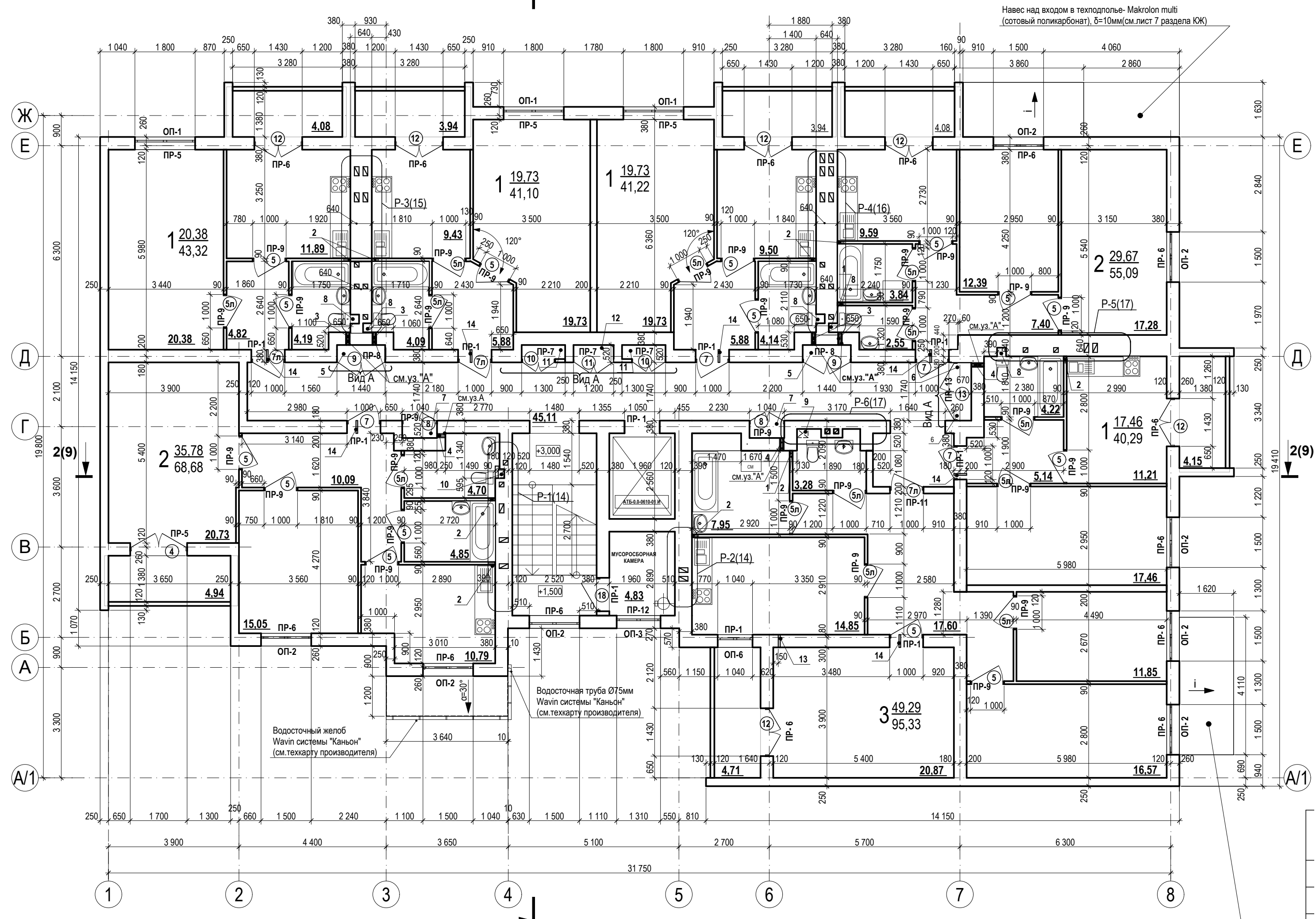
1(8) План типового этажа
