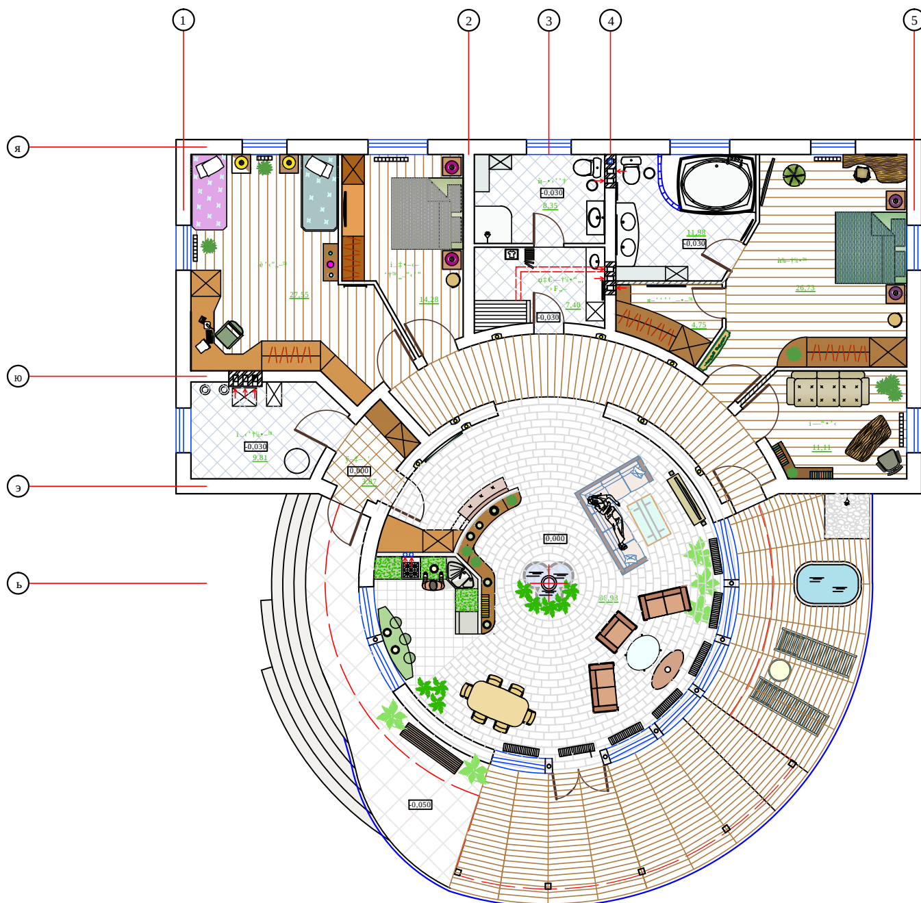
План жилого дома на отм. 0,000
